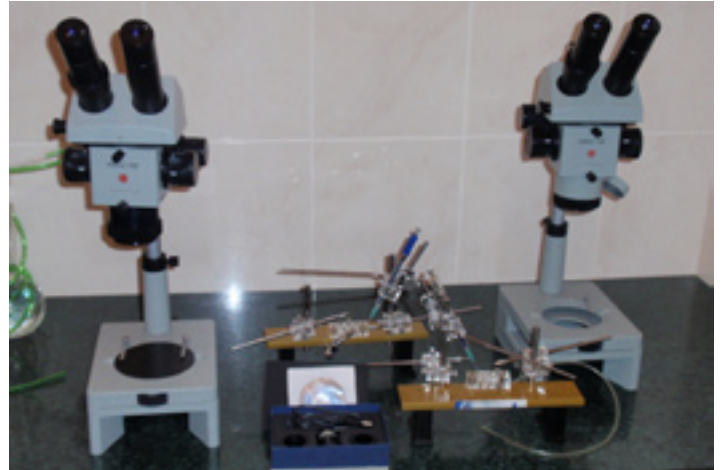
Aparat i mikroskop do inseminacji matek pszczelich.
